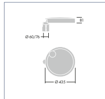
CARAT S MASTAUFSATZ Ø 60 UND Ø 76
