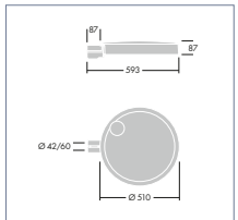
CARAT L SEITLICHE BEFESTIGUNG Ø 42 UND Ø 60
