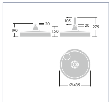
CARAT S HÄNGEBEFESTIGUNG
