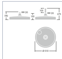
CARAT L HÄNGEBEFESTIGUNG
